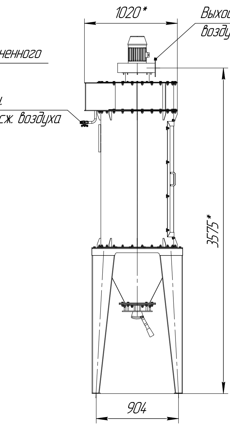
Б(1:10)
