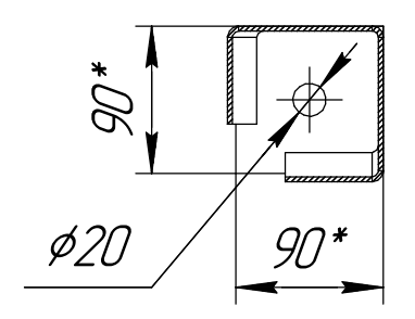
В-В(1:5) 4 места
