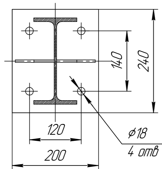
В-В(1:5) 14 мест
