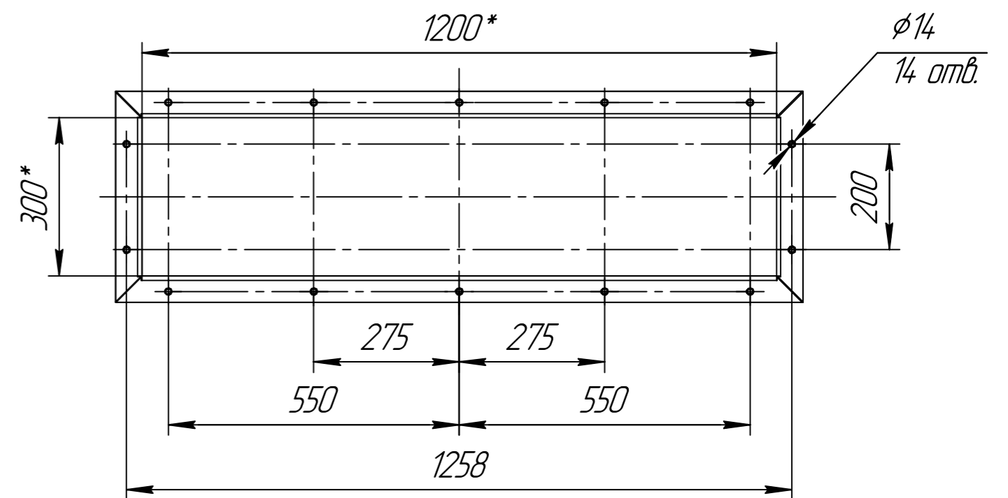
А,Б(1:10)
