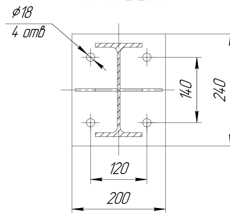
В-В(1:5) 14 мест
