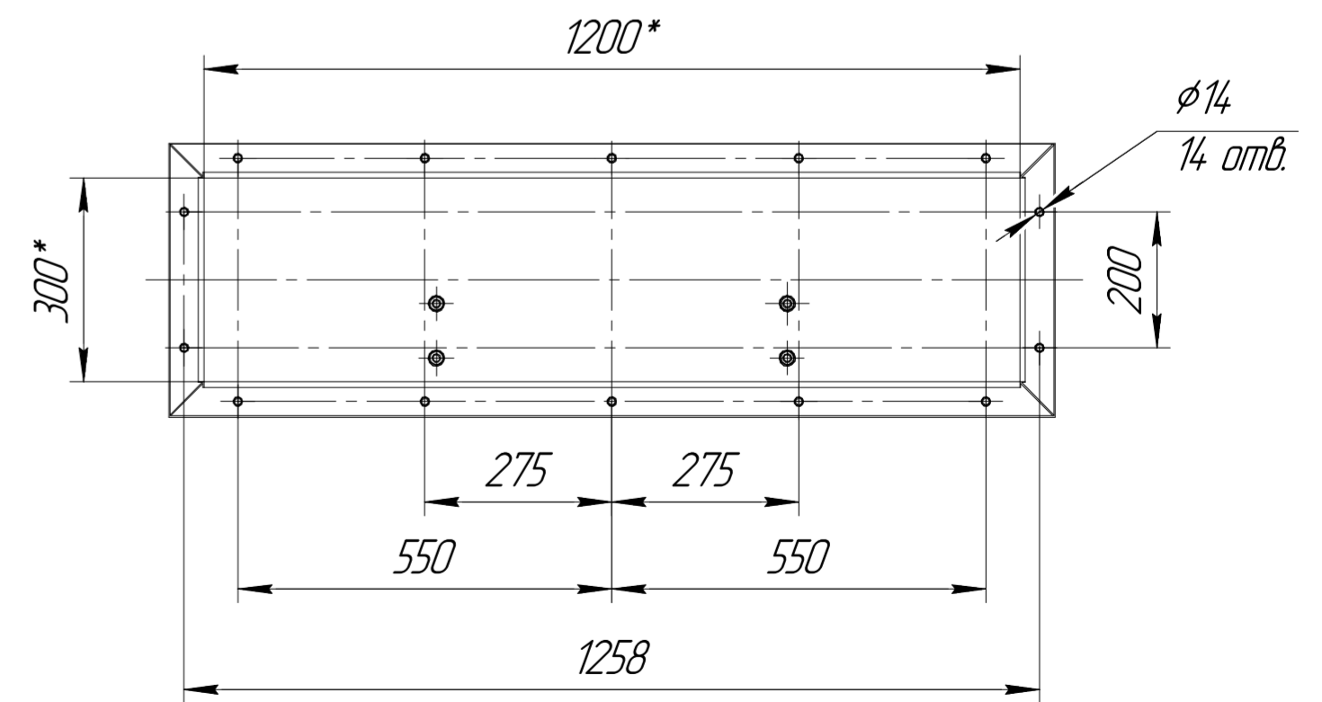
А,Б(1:10)
